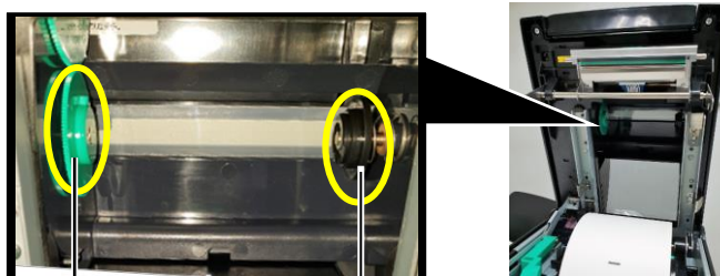
碳帶保持器（供給側）
